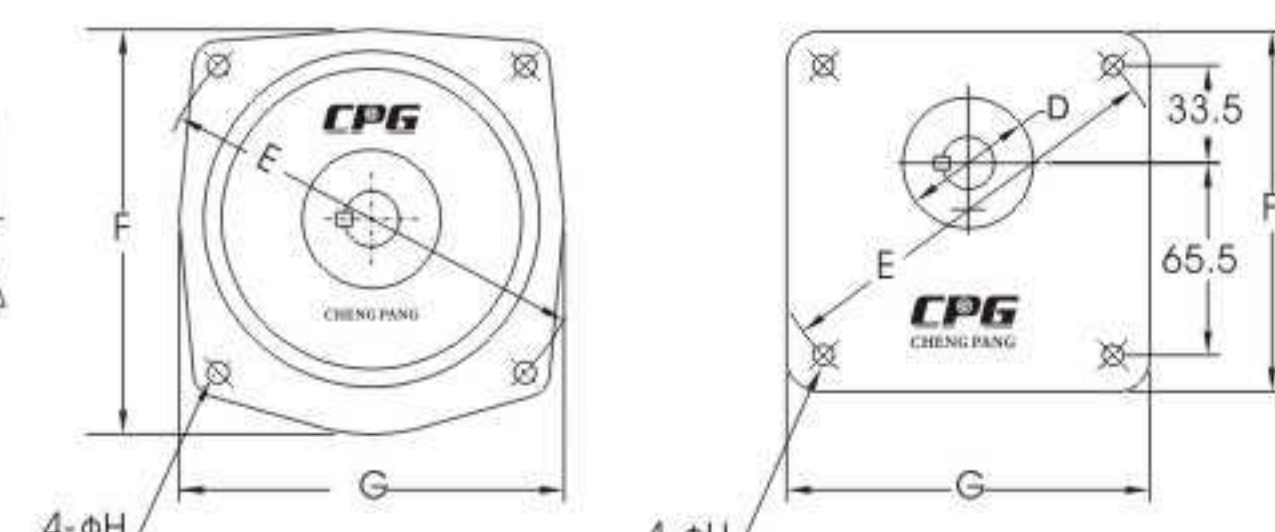
B型法蘭 B TYPE FLANGE
