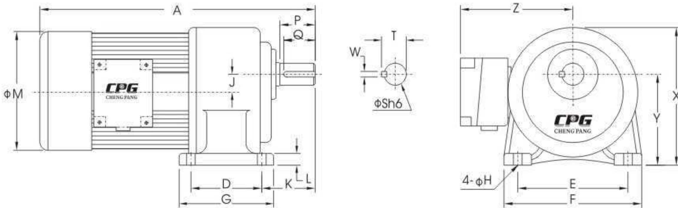
臥式附三相 HORIZONTAL TYPE
