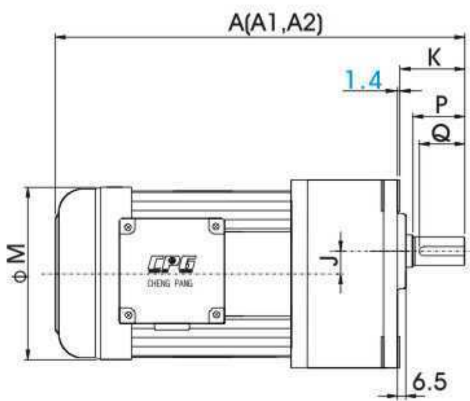
出力軸尺寸 OUTPUT SHAFT
