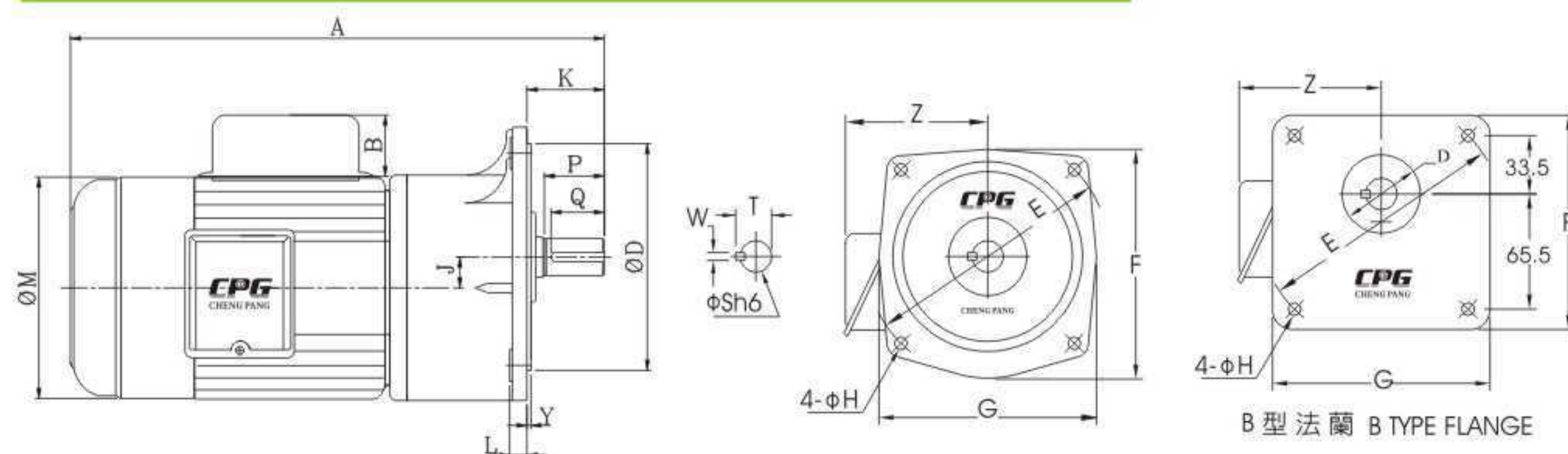
出力軸尺寸 OUTPUT SHAFT
